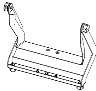
Z5056 M4 Flying bracket
